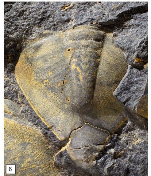
6 : Megistaspis (Ekeraspis) filacovi filacovi
