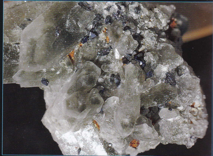
Minéral du groupe de la crichtonite - Cristaux : 2 mm La Fée, les Deux-Alpes, Mont-de-Lans, Oisans, Isère Coll. et photo : S. Vein
