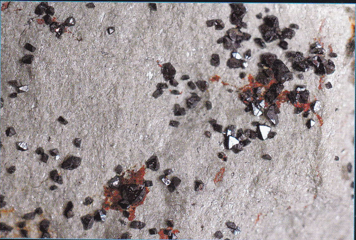
Minéral du groupe de la crichtonite - 4,5 x 4,5 mm La Fée, les Deux-Alpes, Mont-de-Lans, Oisans, Isère Coll. : E. Asselborn - Photo : L.-D. Bayle
