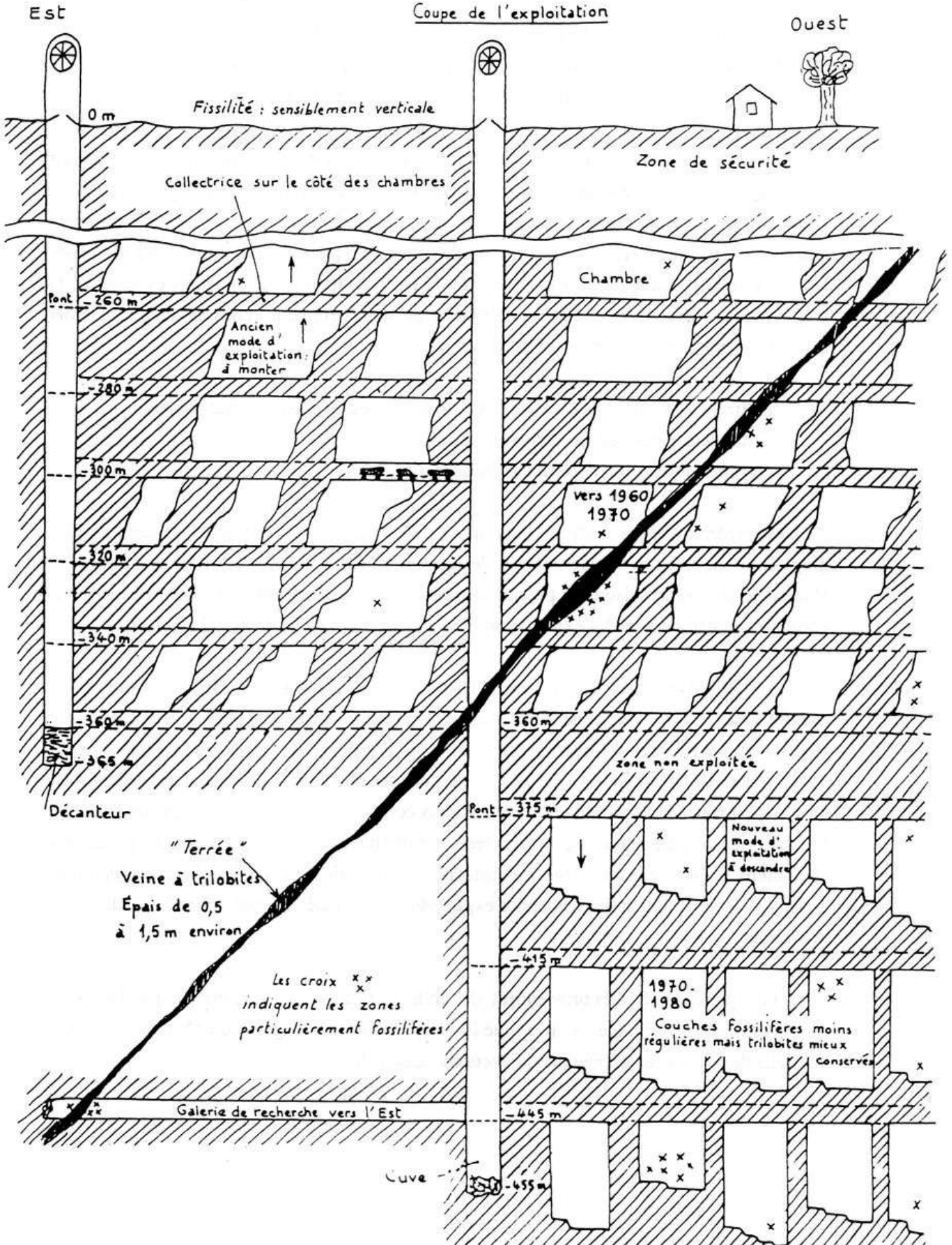
Fig. 3 .- Coupe schématique d'une exploitation d'ardoises de la Pouéze . Cette coupe est due à Mr . Galand et a été recueillie par Mr.Mornand .
