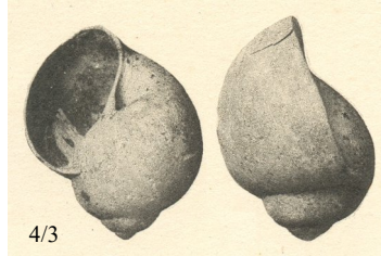
61 - 27 Euspira venusta
