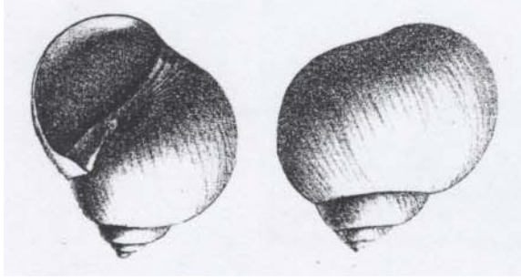
61 - 28 Euspira tenuicula
