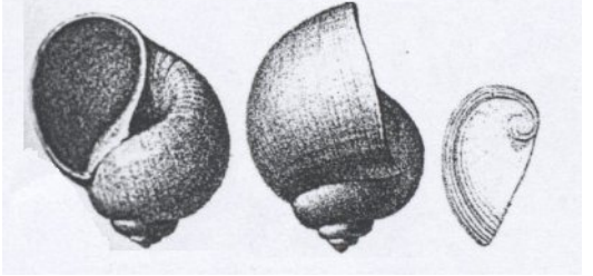
61 - 27 Euspira venusta
