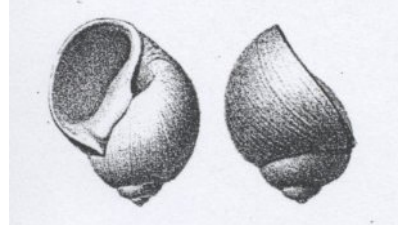
61 - 14 Amauropsina canaliculata
