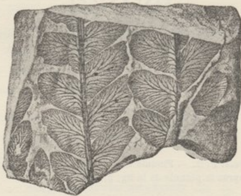
FIG. 8. — Odontopteris Jeanpauli P. B. D'après la figure originale de Potonié.
