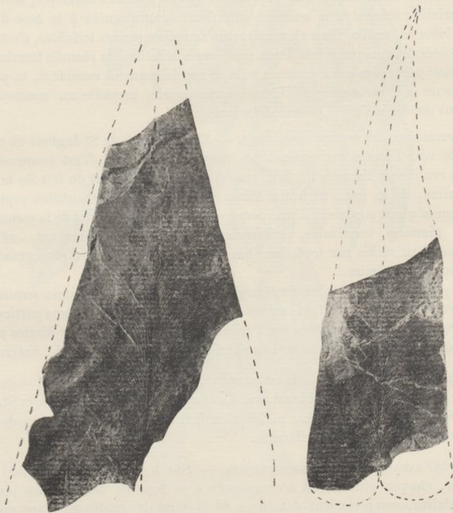
FIG. 2. — Neuropteris Scheuchzeri , var. major . Fragments de pinnules. — Gr. = 1,5 ORIGINE : La Houve, veine Théodore.
