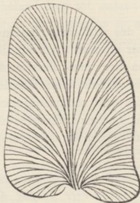
FIG. 6. — Mixoneura Simoni P. B. — Pinnule typique, avec les deux renflements à la base. Parcours nervuraire très schématisé, donc pas très exact (comparer fig. 4 a , Pl. XXIX).
