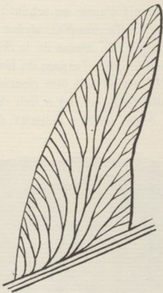
FIG. 7. — Odontopterus Barroisi P. B. — Pinnule montrant la disposition générale des nervures. Croquis exécuté à main levée, d'après la pinnule de la fig. 2, Pl. XXX.
