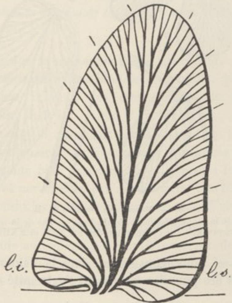
FIG. 4. — Mixoneura Destinei P. B.
