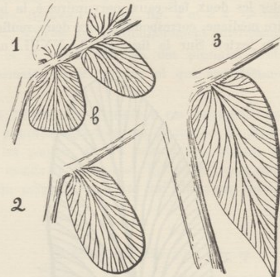
FIG. 5. — Mixoneura Deflinei P. B. Variations de forme de la pinnule basilaire, b , du haut en bas de la même penne primaire (croquis pris sur l'échantillon des Pl. XXII et XXIII).
